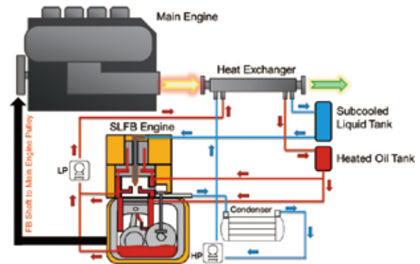
蒸気機関 (SLFB Engine)
